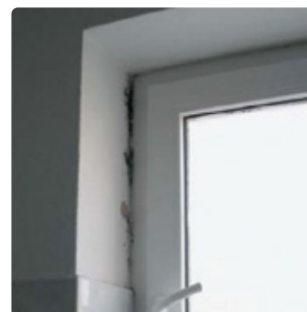
Condensações e desenvolvimento de fungos no lado interior
