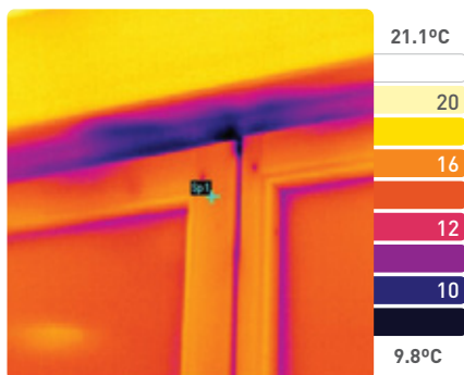
Entrada de ar frio para o interior
